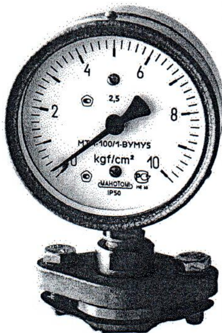
Рисунок 1 - Фотография общего вида приборов
