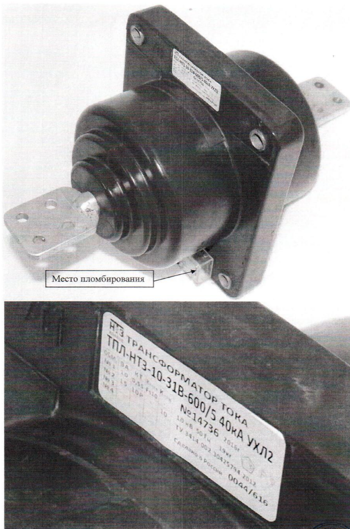
Рисунок 1 - Общий вид трансформаторов тока ТПЛ-НТЗ
