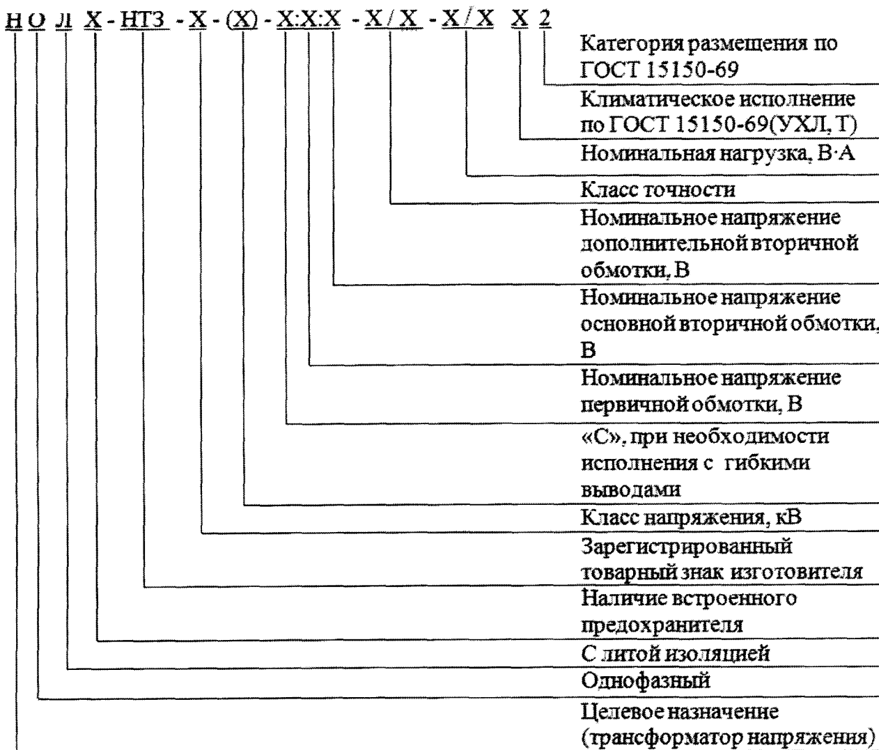
Рисунок 3 - Структура условного обозначения трансформаторов напряжения НОЛ(П)-НТЗ
