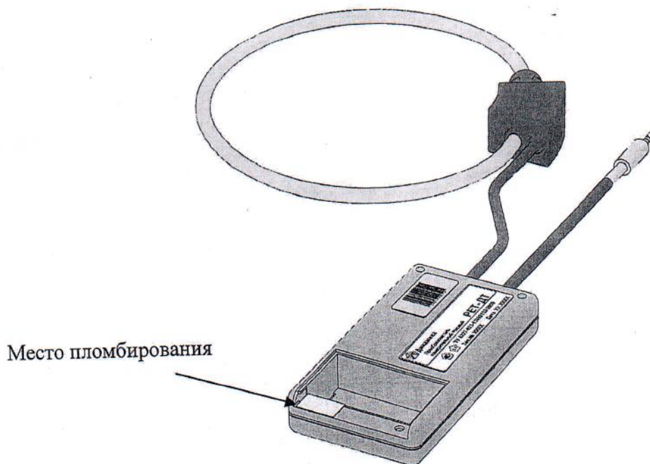
Рис. 2 – Внешний вид преобразователя измерительного токового РЕТ-ДТ сзаци (без крышки батарейного отсека)
