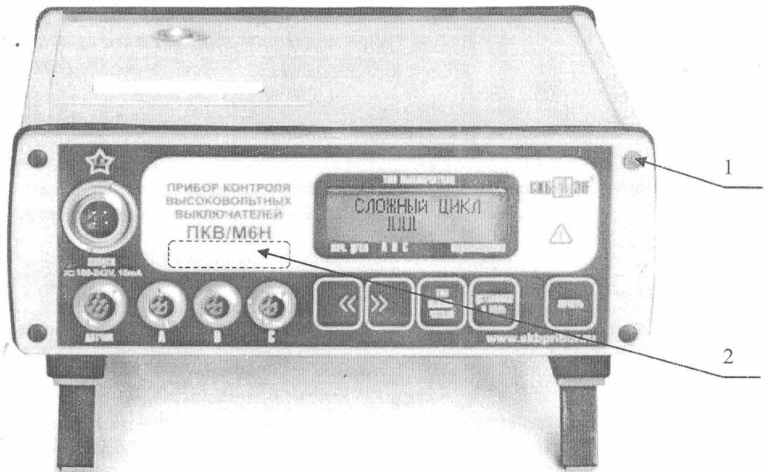
Рисунок 1 - Измерительный блок ПКВ/М6Н
