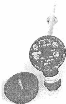
Рисунок 4 - Общий вид ДТП модификации XX5 со встроенным нормирующим преобразователем
