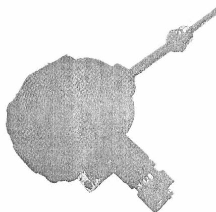
Рисунок 3 - Общий вид ДТП с клеммными головками модификации XX5
