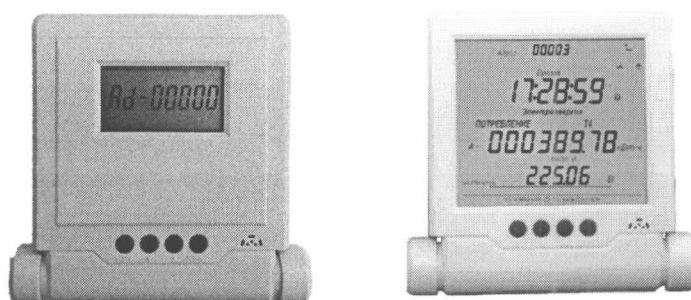
Рисунок 3 - Внешний вид выносных модулей отображения информации.
