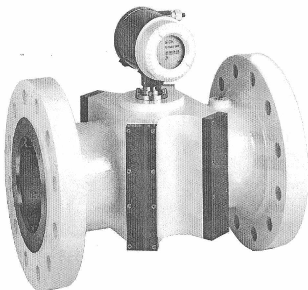
Расходомер ультразвуковой FLOWSIC600
