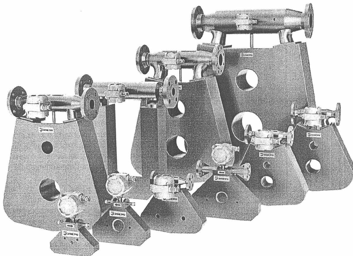
Рисунок 1 - Датчики расходомера
