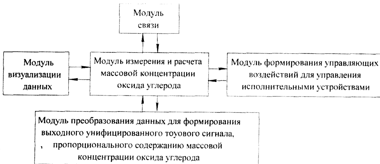
Рисунок 3 - Структура ПО
