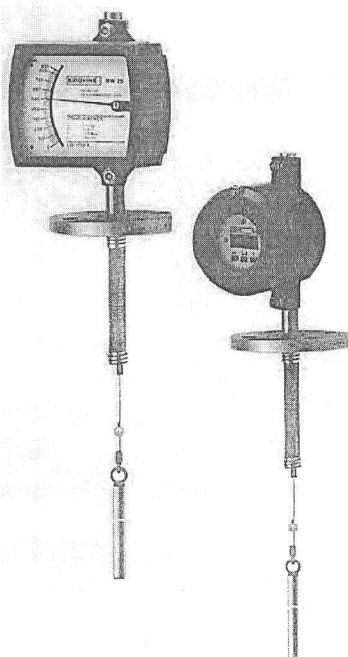
Рисунок 1 - Внешний вид уровнемеров буйковых BW 25
