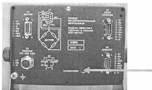
Рисунок 2 - Места пломбирования терминала М0601 для нанесения знака поверки
