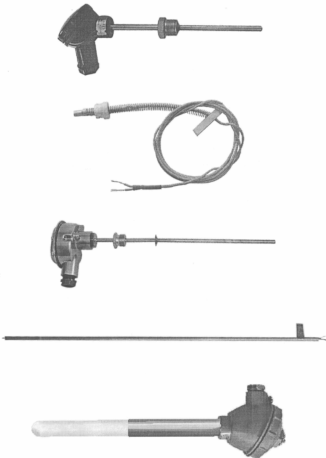
Рисунок 1 – Внешний вид преобразователей термоэлектрических ТХА(К)-1199, ТХК(Л)-1199, ТЖК(Ј)-1199, ТНН(Н)-1199, ТПП(С)-1199, ТПП(R)-1199, ТПР(В)-1199
