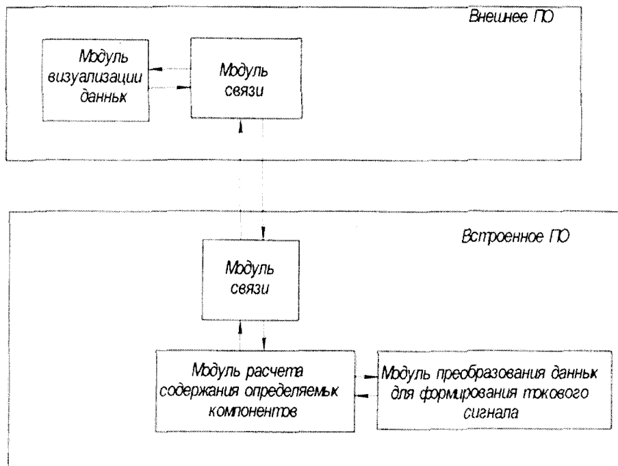
Рисунок 5 - Структура ПО.
