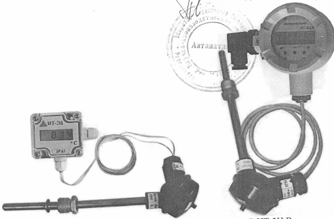
а) ИТ-2Ц
