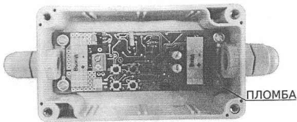
в) Плата преобразователей ИТ-2.хД (крышка снята)
