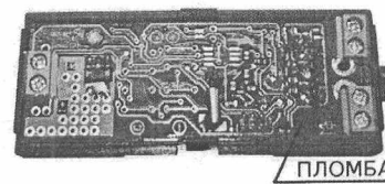
г) Плата преобразователей ИТ-2.хР (крышка снята)
