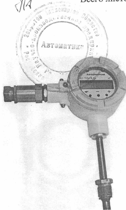
в) ИТ-1ЦМ.В-Ex
