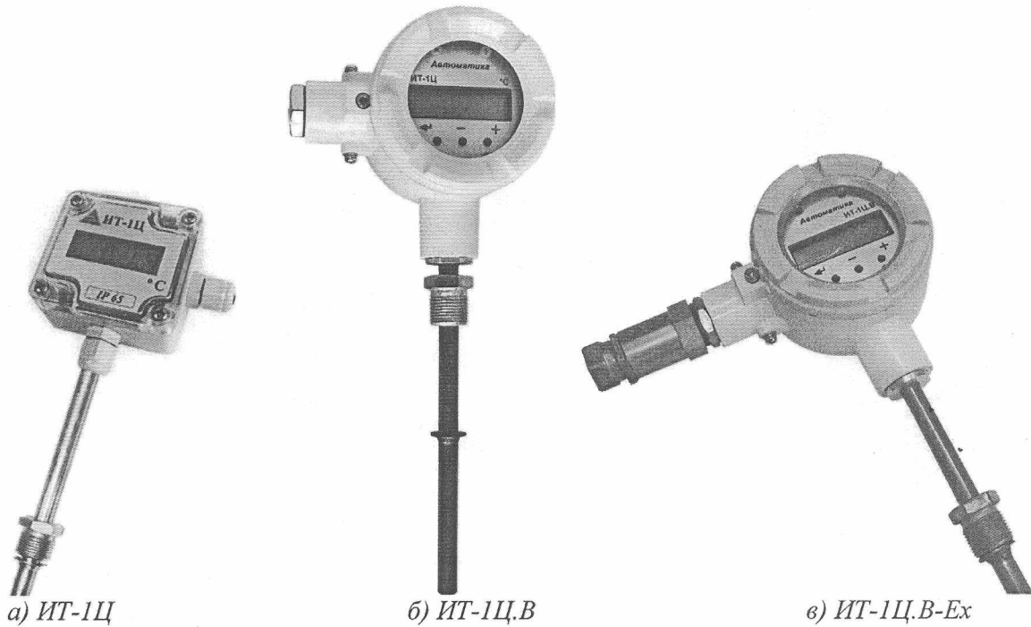
Рисунок 2 – Термопреобразователи ИТ-1Ц, ИТ-1Ц.В, ИТ-1Ц.В-Ex
