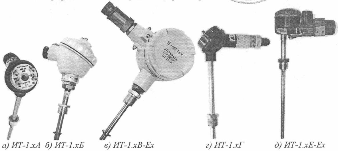
Рисунок 1 – Термопреобразователи ИТ-1.хА, ИТ-1.хБ, ИТ-1.хВ, ИТ-1.хГ, ИТ-1.хЕ
