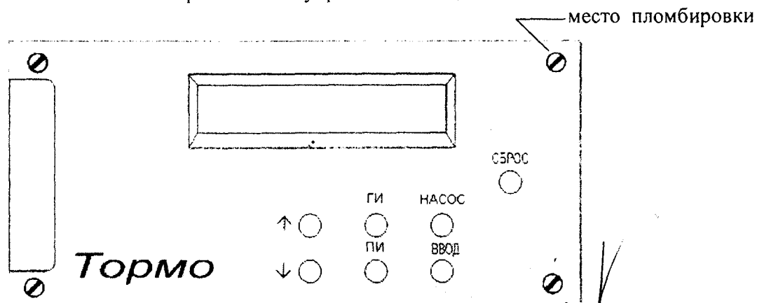
Схема пломбировки блока управления стенда СИЗР
