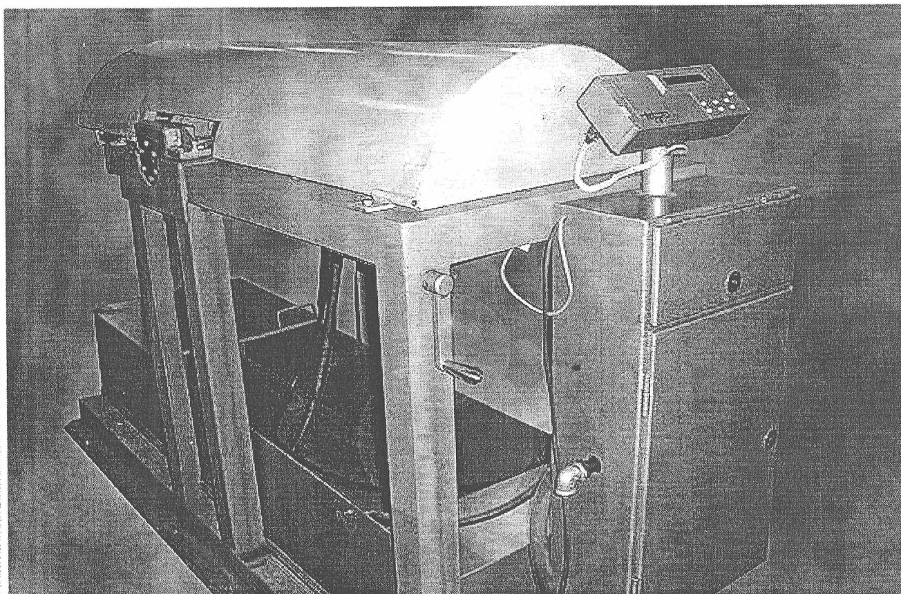
Фотография общего вида стенда СИЗР
