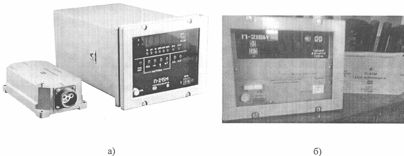
Рисунок 1 – Общий вид преобразователей а) П-215М; б) П-215И
