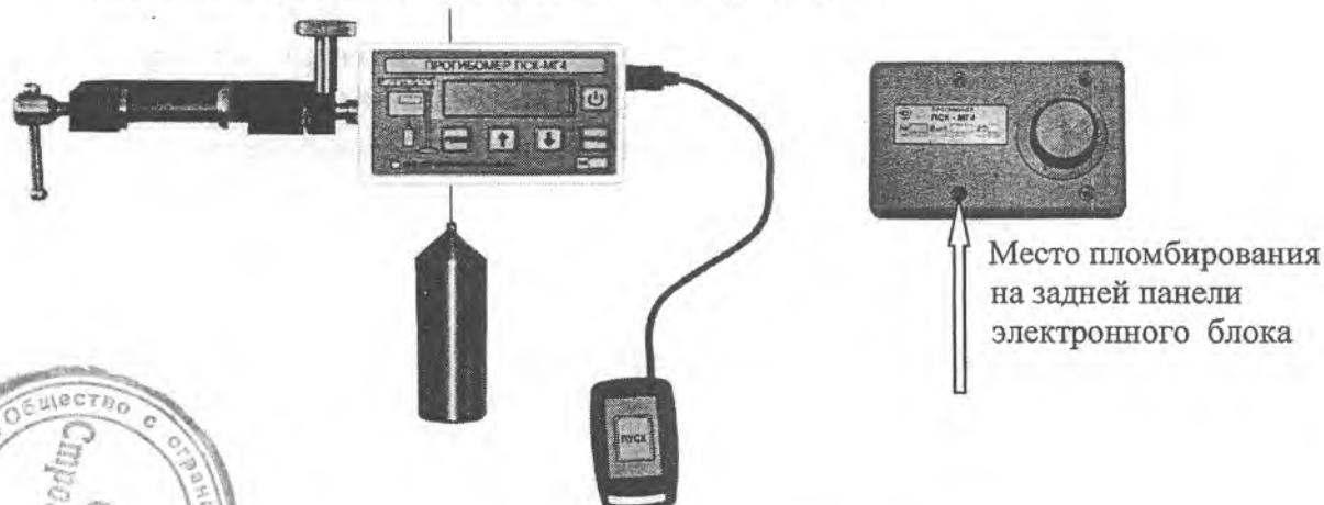
Рисунок 1 – Общий вид прогибомера
