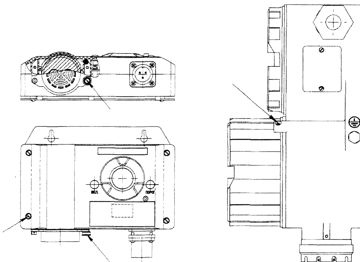
а) ДАТ-М-01/-02/-03/-04
