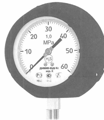
Рисунок 10 – Приборы кислотостойкие
