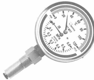
Рисунок 8 – Манометр МПТ с функцией измерения температуры
