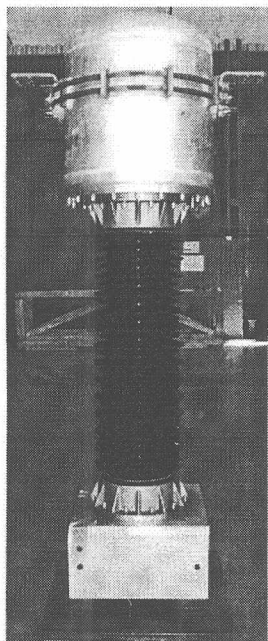
Рисунок 1. Общий вид трансформатора тока ТОГФ-110
